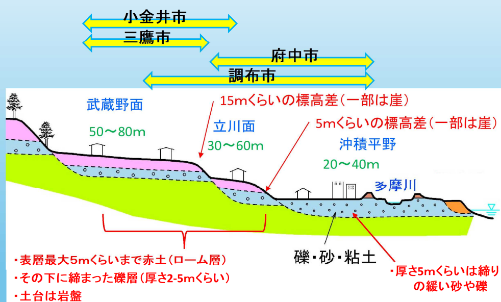
調布／府中／三鷹／小金井周辺を模式的に示した地質断面図
