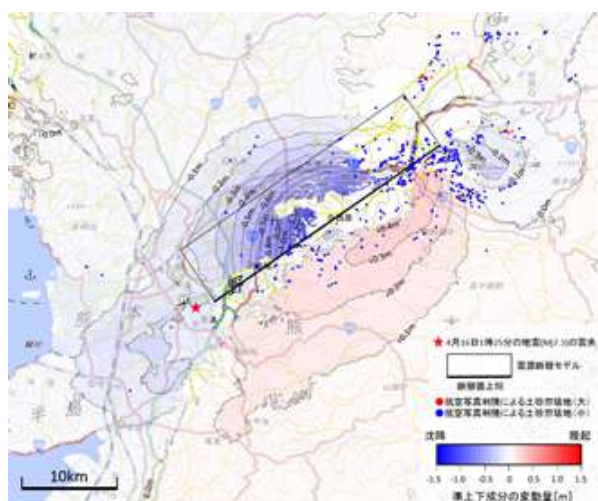
図-1 2.5 次元解析による準上下成分算出結果
