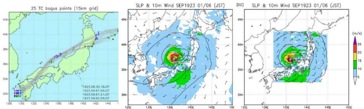
図2：数値シミュレーションの結果。左：複数の台風経路。初期位置を変えた25メンバーによる台風経路の結果。中と右：9月1日6時における代表的な風向（矢羽根）と地上風速（色）と海面高度気圧（線）。中が親領域、右が子領域。
