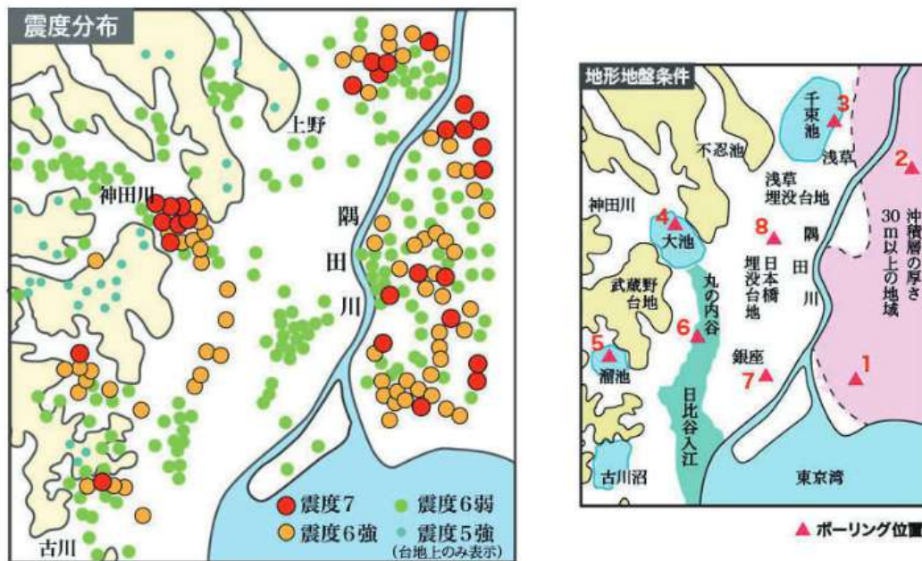
図1 関東地震における東京の震度分布と地形・地盤条件 (防災科学技術研究所 HP「防災基礎講座：地域災害環境編」より引用)
