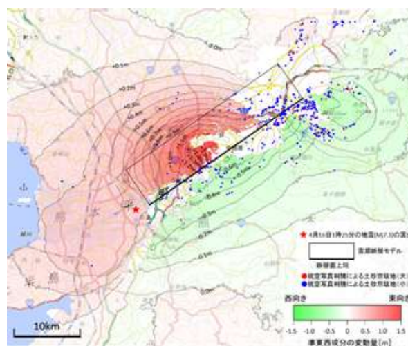
図-2 2.5 次元解析による準東西成分算出結果
