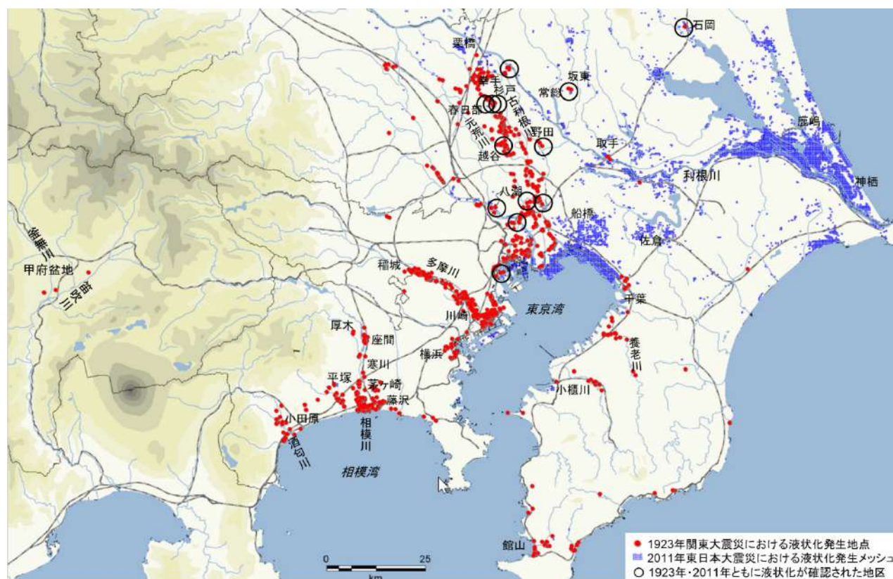
図1 1923年関東大震災と2011年東日本大震災における液状化発生地点
