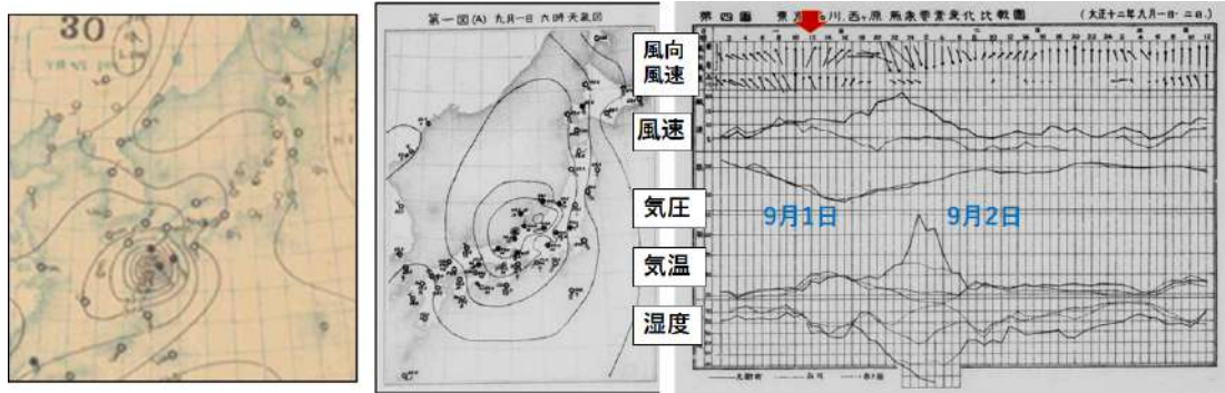
図1：中央気象台作成の解析天気図と中央気象台（東京）と品川の地上観測結果。左から1923年8月30日18時の解析天気図、9月1日06時の解析天気図、9月1日00時～3日12時の地上観測データの表示（赤い矢印は地震発生時刻）。
