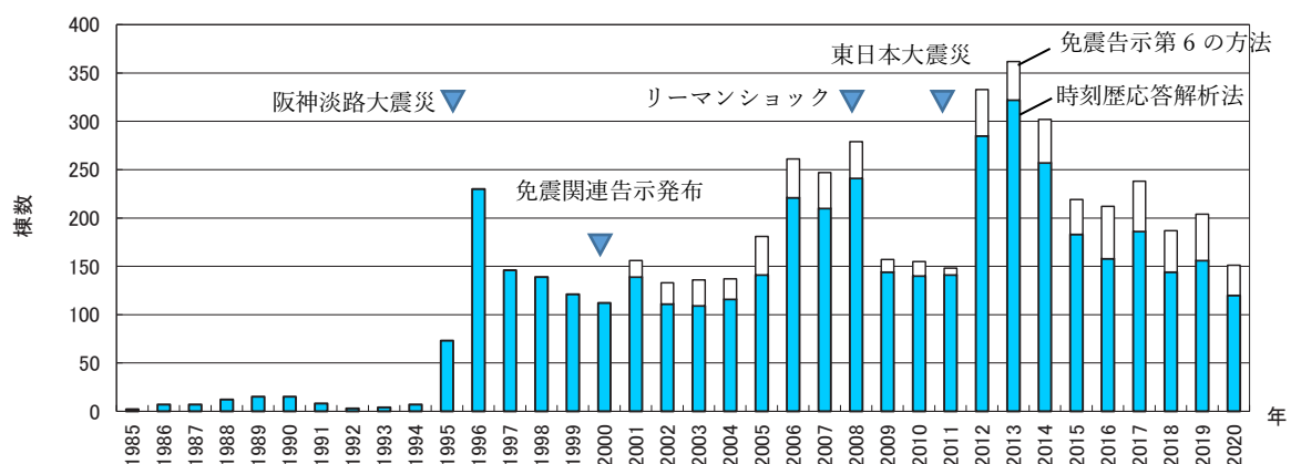
図1 免震建築物の計画推移
