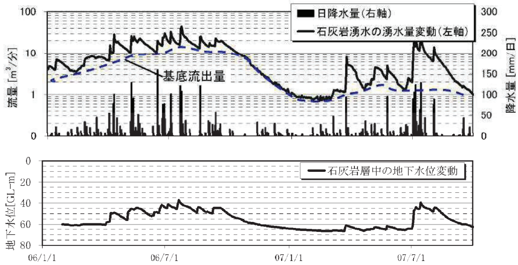
図-4 石灰岩地帯における地下水位観測孔の水位変動と近接する湧水地点の湧水量の変化の事例 5)
