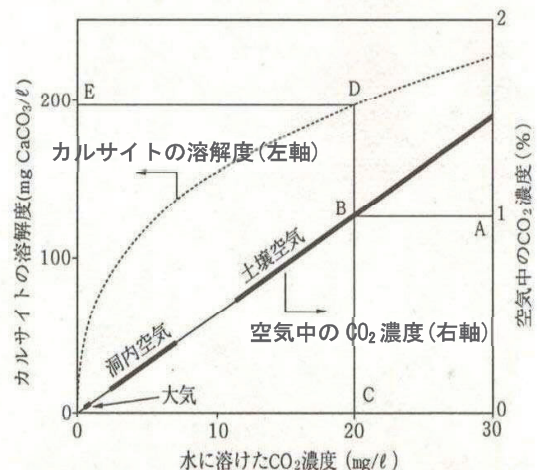
図-1 石灰岩の溶解に及ぼす二酸化炭素濃度の効果 2)
