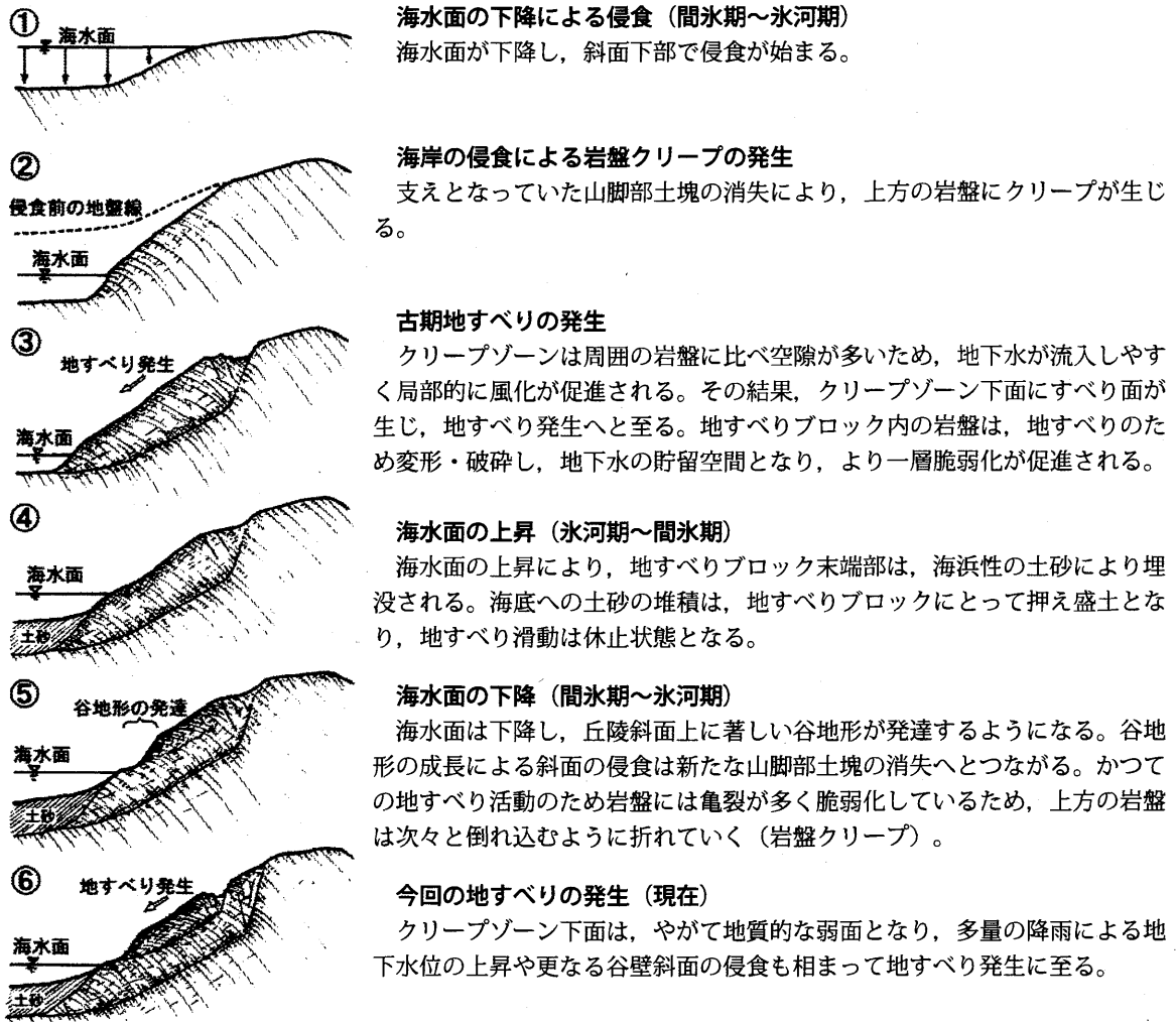
図-5 当該箇所の地形形成史模式図
