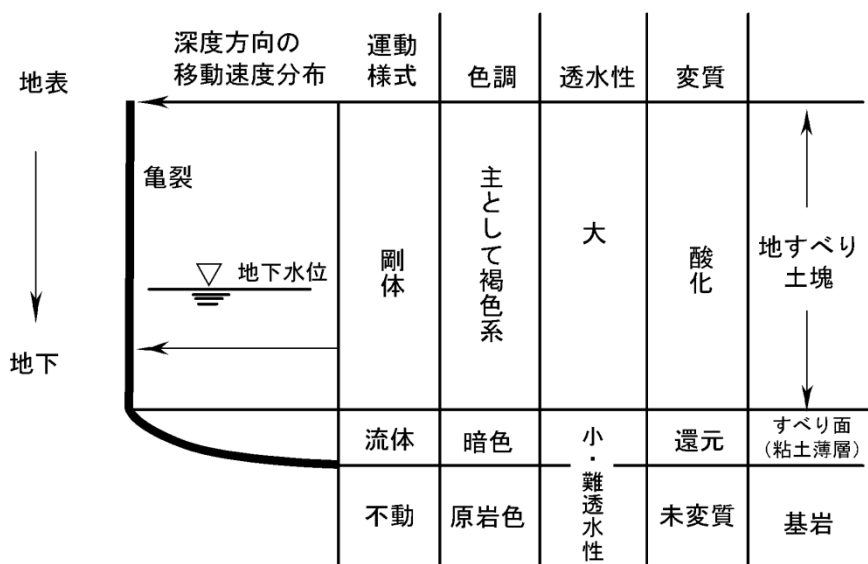
図-3 地すべり斜面の構成 4)
