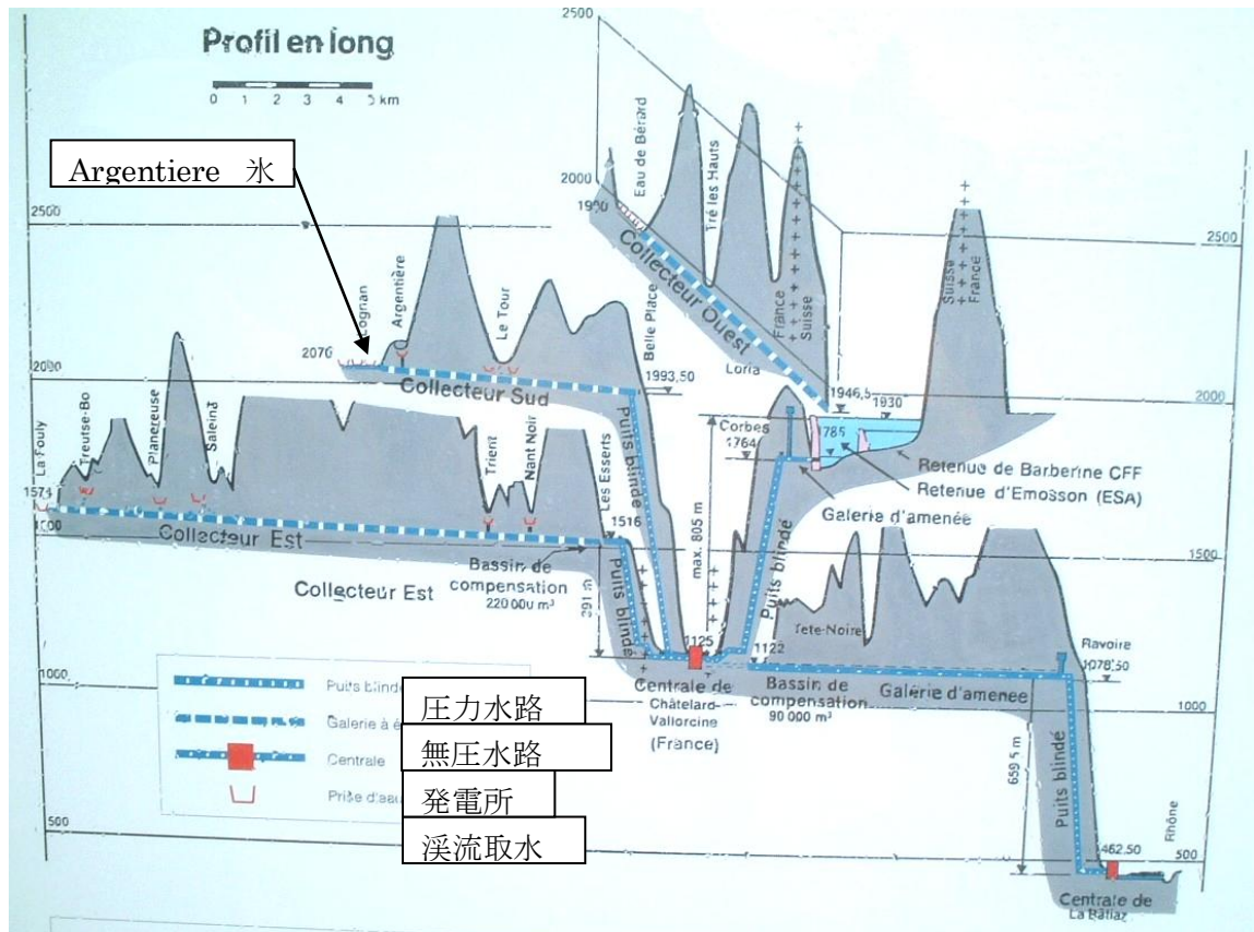
図-2 エモッソンドムの水力発電にかかる模式縦断面図
