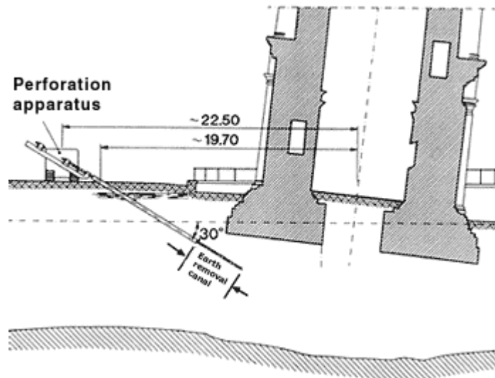
図-6 オーガーによる排土工
