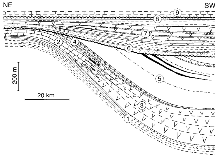
図6 シチリアのメシニアン階の地層断面模式図(Decima と Wezel,1973 の加筆)
