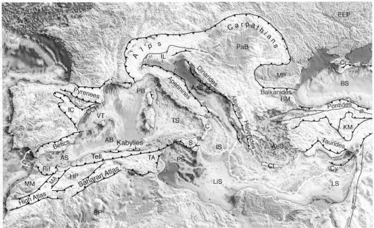
図1 地中海域の主要、かつ単純化した地質構造と地形モデル。白いスラスト記号はイオニア海と東地中海のもぐり込み帯沿いの外側の変形フロントを示す。
