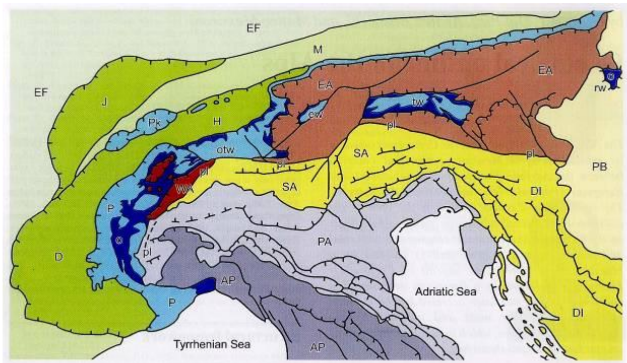
図1 アルプスの構造図—(1)ヨーロッパ衝突帯：i)西部(WA)と東部(EA)オーストリアアルプス；ii)ペンニン域：西アルプス軸(P)の大陸性やオフィオライト(o)ナップ群(otw：Ossola-Ticino,ew:Engadine,tw:Tauern,rw:Rechnitz)；プレアルプスクリッペ(Pk)；iii)ヘルベット-Dauphinois(H-D)域；iv)モラッセ沈降盆(M)；v)ジュラ帯(J)。(2)南アルプス(SA)、Periadriatic 構造線(pl)で北を境される。パノニアン盆地(PB)、ヨーロッパ(EF)とポー平野・アドリア(PA)前縁地、ジナル(DI)とアペニン(AP)のスラスト・褶曲地帯
