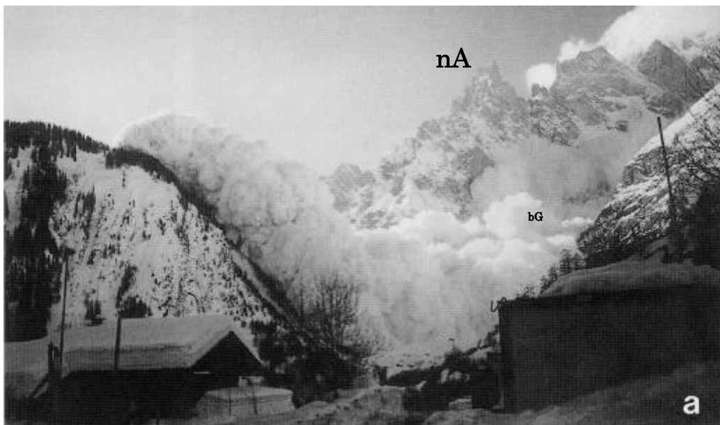
写真-2 1997年1月18日発生の岩なだれで引き起こされた、Veni谷の対岸斜面を 90 渡る雪煙なだれ(airborne powder avalanche)。(文献1からの引用)
