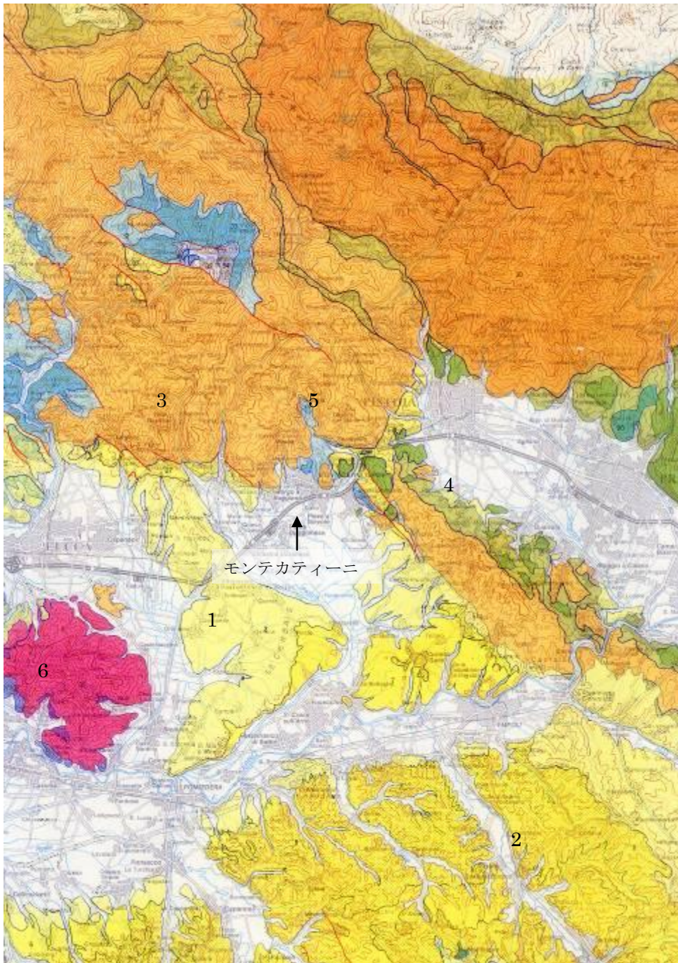
モンテカティーニ周辺域の地質図(IGC 資料 ; Geological Map of TUSCANY, 2004) 地質凡例 ; 1;第四紀陸成層、2;第四紀海成層、3;非変成フリッシュ層、4;白亜紀・暁新世堆積岩類、 5;前期白亜紀-漸新世
