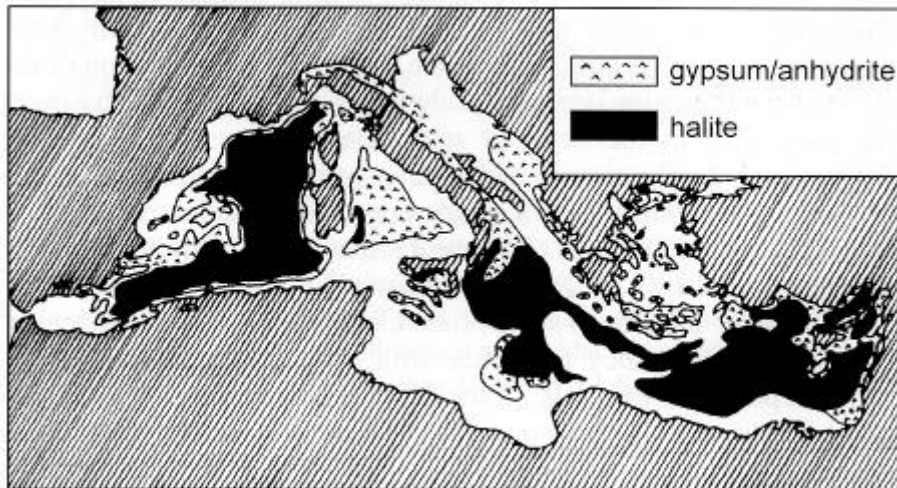
図 5 地中海域におけるメシニアン階の蒸発岩類の広がり。Rouchy(1980)に加筆
