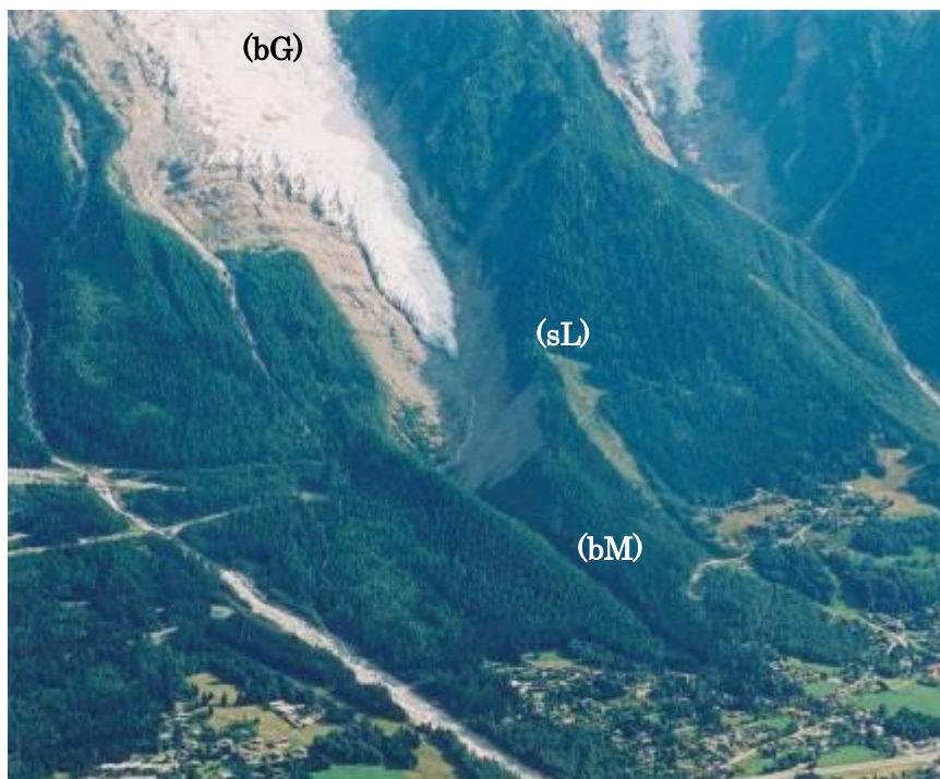
写真一 2 ボソン氷河(bG)の氷舌端とモレーン丘(bM)
