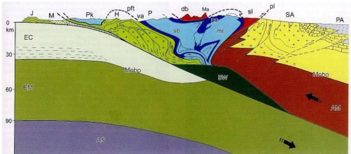
図 2 北から西部アルプスの地殻断面－1)オーストリアアルプス：Sesia-Lanzo(sl)とDentBlanche ナップ群(db)、マッターホルン(Ma)を含む；2)ペンニン帯(P)：Piedmont オフィオライトユニット(po)、ペンニン下部とペンニン外帯の Valais 帯(va)を覆う MonteRosa(mr)と GrandSt.Bernard(sb)ナップ群、ペンニンクリップ(pk)、ペンニン前面のスラスト(pft)；3)ヘルベッティ帯の基盤スライスとカバーナップ群(H)；4)モラッセ沈降盆(M)；5)ジュラ帯(J)；6)ヨーロッパマントルまたはエクロジヤイト化した地殻ユニットの隠れた楔(BW)；7)ヨーロッパリソスフェア：大陸地殻(EC)とマントル(EM)；アセノスフェア(AS)；8)アドリアリソスフェア：南アルプス(SA)とマントル(AM)；Periadriatic 構造線(pl)；9)Padane-アドリア前縁地(PA)
