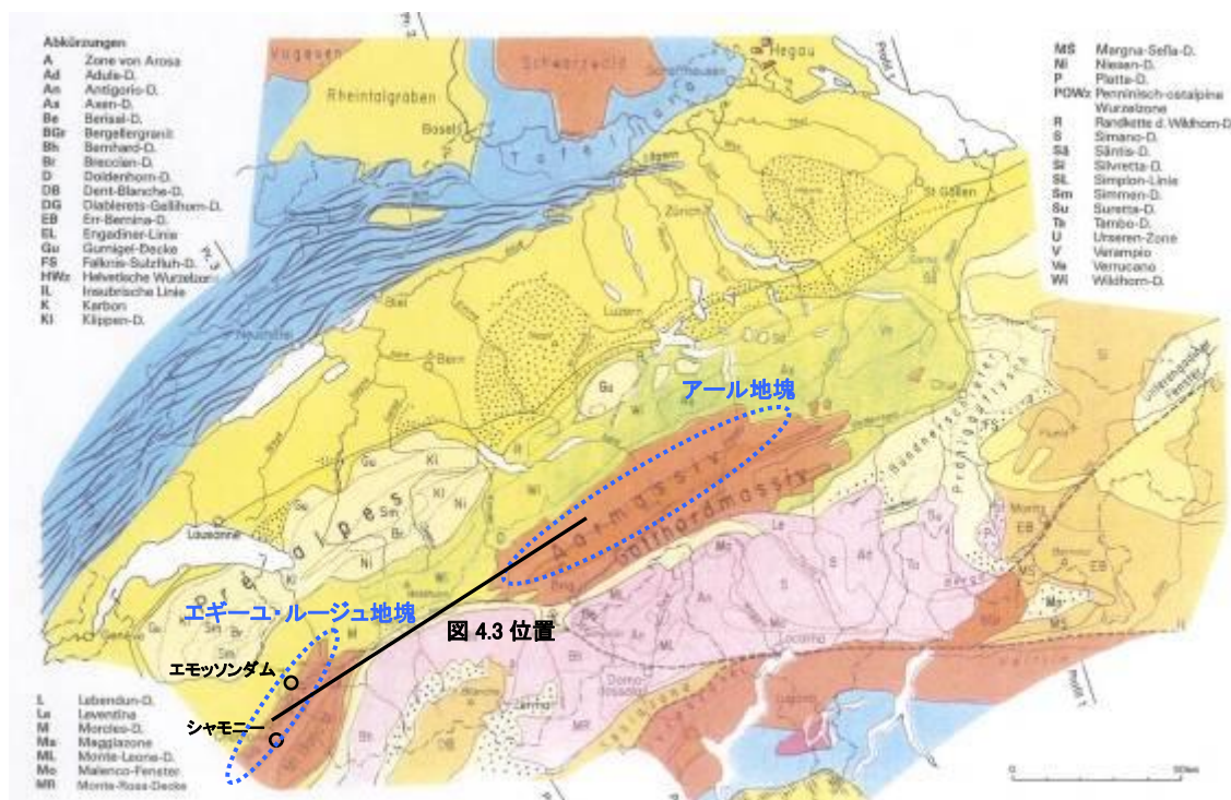
図 1.1 アルプスの地質
