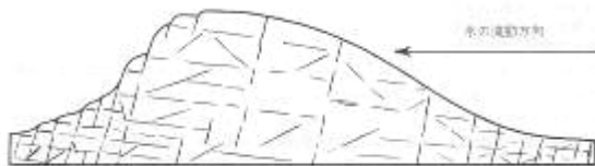
図一1 典型的な羊背岩の断面 (A.Homes,1984 より引用)
