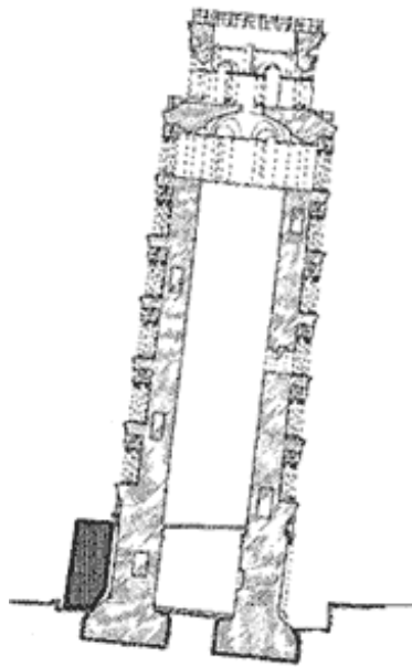
図-3 鉛インゴットによるカウンターウェイト (ピサの斜塔公式サイト(伊)HP)
