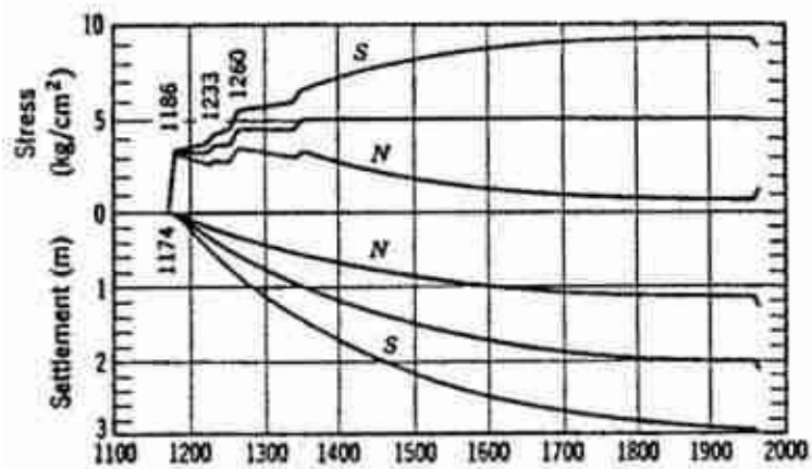
図-1 ピサの斜塔の基礎地盤と沈下状況
