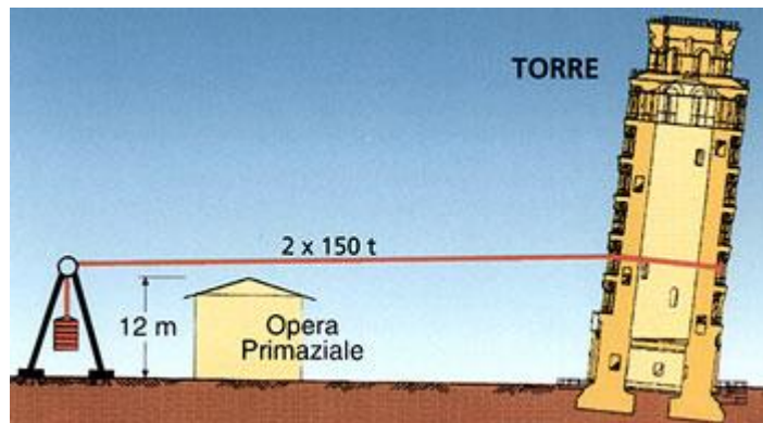
図-4 ステー（支索）による対策 (ピサの斜塔公式サイト(伊)
