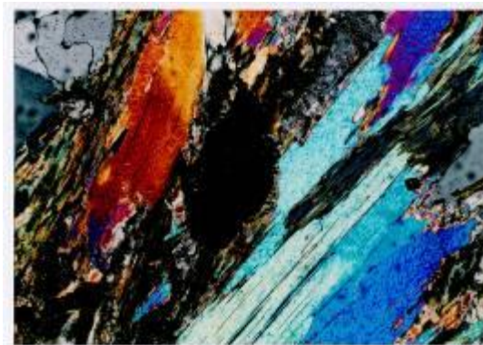
③-2 ×10 クロスニコル
