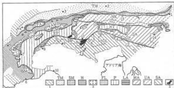
図1.21 アルプス地域のアルプス変動帯。記号TM-SAは図1.22参照。1はジュラ山脈、2は Helvet 帯基盤、3は第三紀カコウ岩類 A: Adamello, AM: Aar 地塊, AR: Aiguilles-Rouges 地塊, DB: Dent-Blanche ナップ, DL: Dolomiten, DZ: Drauzug, EN: Unterengadiner Fenster, GA: Gurtal-Alpen, GL: Gail 嶺, GM: Gottard 地塊, HT: Hohe Tauern, IL: Insubric 帯, JL: Judicarie 嶺, KA: Karnische Alpen, LEP: Lepontina, MM: Mont Blanc 地塊, NG: 北 Grauwacke 帯, NK: 北 Kalkalpen(北石灰アルプス), PA: Préalpes, SB: 南アルプス先中生代の基盤, SZ: Sesia-Lanzo 帯, TV: Taverisch 中間地塊, W: Wechselfenster 1: Wien, 2: München, 3: Zurich, 4: Genève, 5: Grenoble, 6: Nice, 7: Briançon, 8: Ivrea, 9: Como, 10: Genova, 11: Tonal 峠, 12: Innsbruck, 13: Salzburg, 14: Graz
