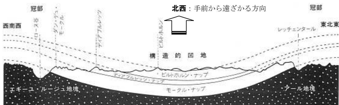
図 4.3 エギーユ・ルージュ地塊－アール地塊の模式断面図 (図 1.1 参照)
