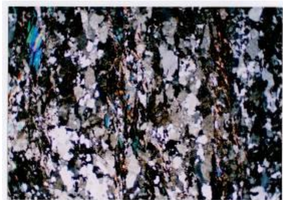
③-1 ×1 クロスニコル
