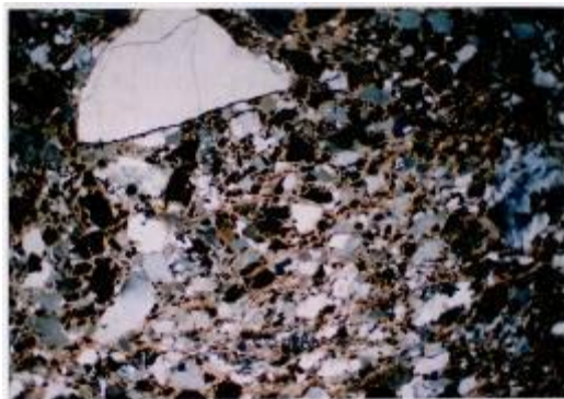
④-1 ×1 クロスニコル
