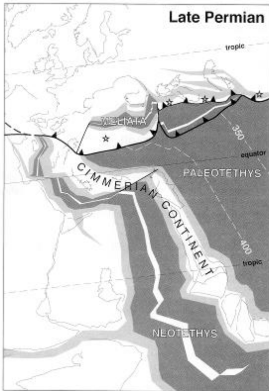
図2 後期二畳紀における西部テチス海域の古地理復元図(Stampfli ら,2001,若干加筆)。星印はマグマ活動を示す。
