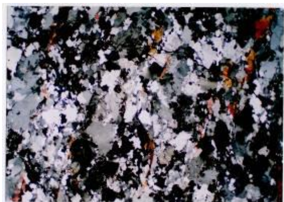
①-1 ×1 クロスニコル
