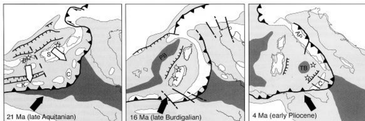
図 4 新第三紀における地中海域の構造発達の様式図(Bonardi ら,2001,Roca,2001 に加筆) 活動する構造要素のみ記入。白、陸地；淡い灰色、大陸縁の海；濃い灰色、海洋地殻；黒い矢印はヨーロッパに対するアフリカの動きを示す(Mazzoli と Helman,1994)。白い矢印は上部プレート の拡大方向を示す。星印はもぐり込みに関係するマグマ活動を示す。
